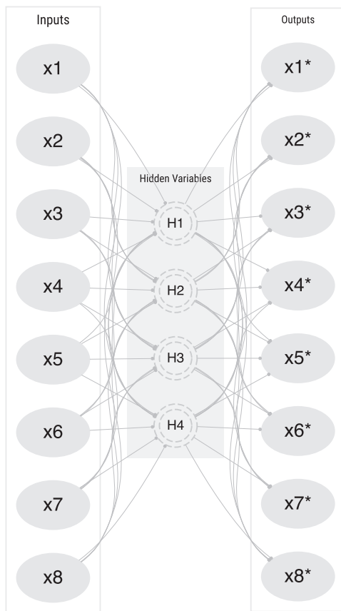
Figure 12.2: PCA or autoencoder.
