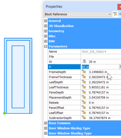
Editing parameters of door
