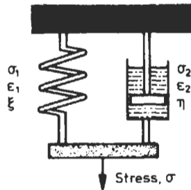
Fig. 2.36 The Kelvin or Voigt Model
