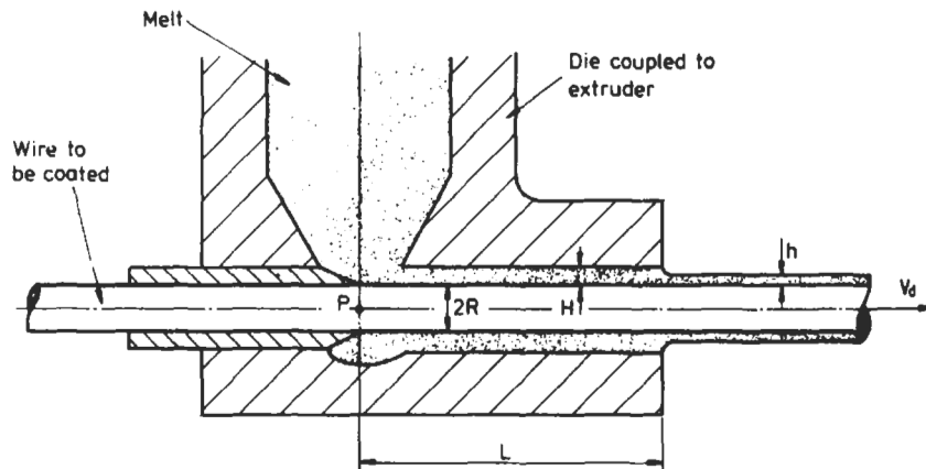
Fig. 4.27 Wire Covering Die
