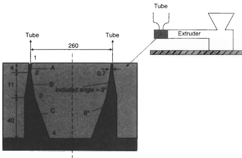
Fig. 5.20 Tube Extrusion Die
